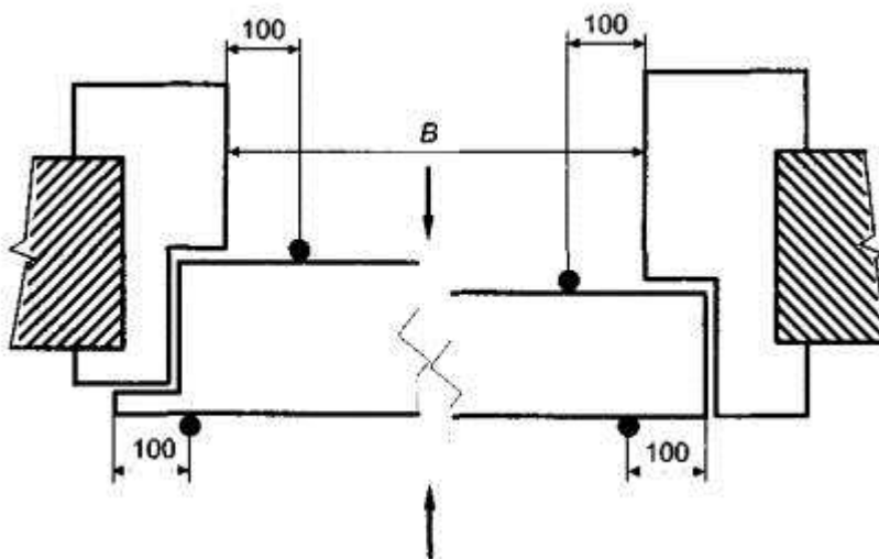
B - ширина проема в свету; \uparrow , \downarrow - вид на необогреваемую поверхность
