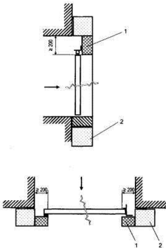
Рисунок 6 - Схемы монтажа образцов распашных дверей (вертикальное сечение)
